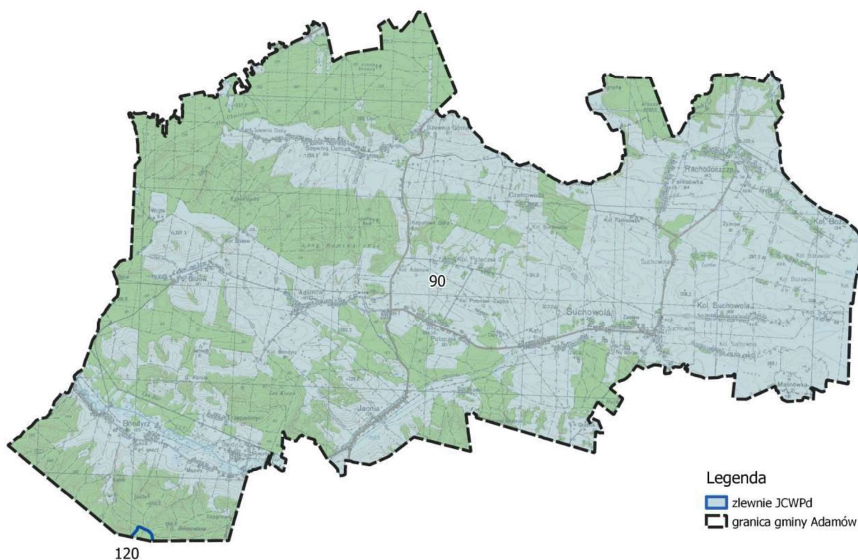
Ryc. 7. Jednolite części wód podziemnych na terenie Gminy Adamów
