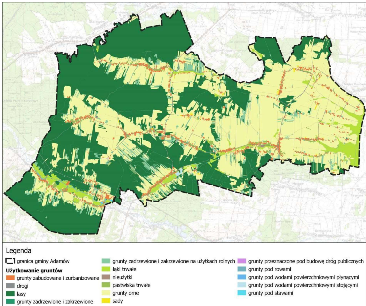
Ryc. 5. Użytkowanie gruntów w Gminie Adamów
