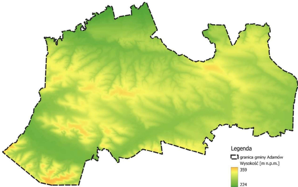
Ryc. 4. Rzeźba terenu Gminy Adamów
